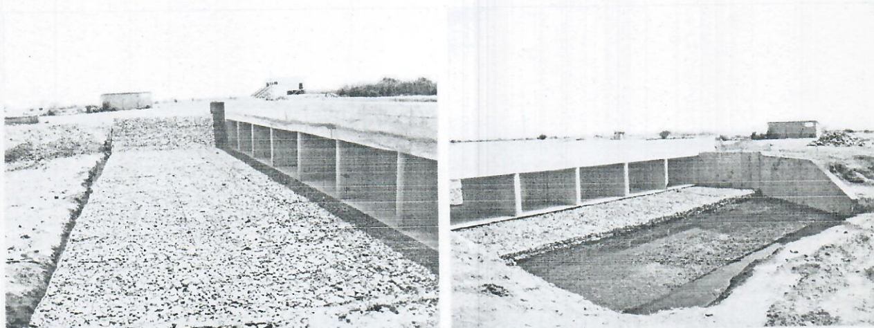
Déversoir de Krankaye en cours de finition
