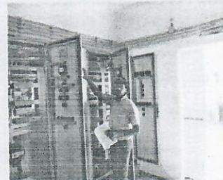
équipements électromécaniques de la station d'irrigation (armoire de commande)
